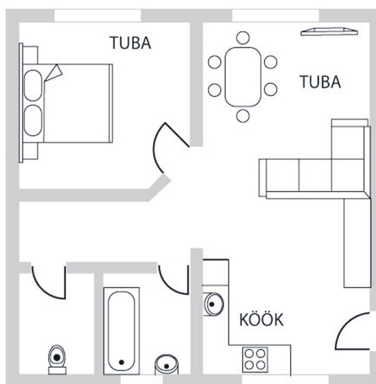
Joonis 6. Korteriplaan
